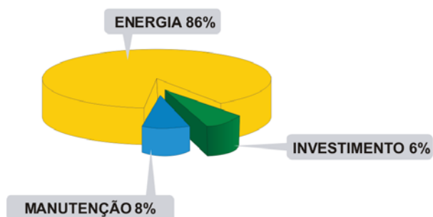
CUSTOS TOTAIS CICLO VIDA COMPRESSOR
